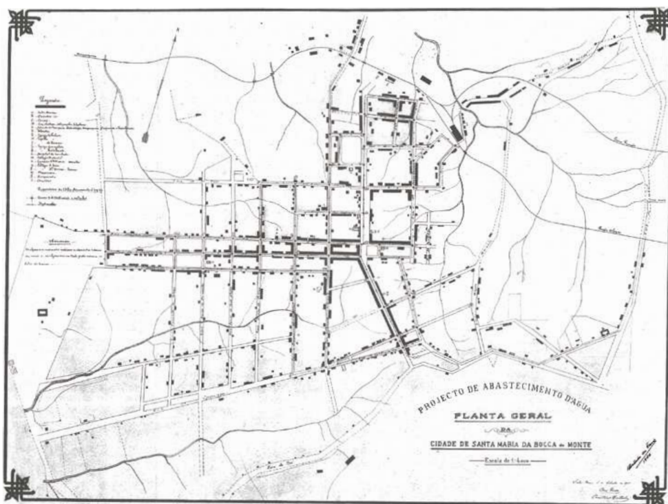
Figura 56: projeto de abastecimento d'água de Santa Maria elaborado e assinado pelo engenheiro Oscar Ewald e pelo desenhista Constant Methelin datado de 01 de setembro de 1905. Fonte: acervo da mapoteca da SOP.
