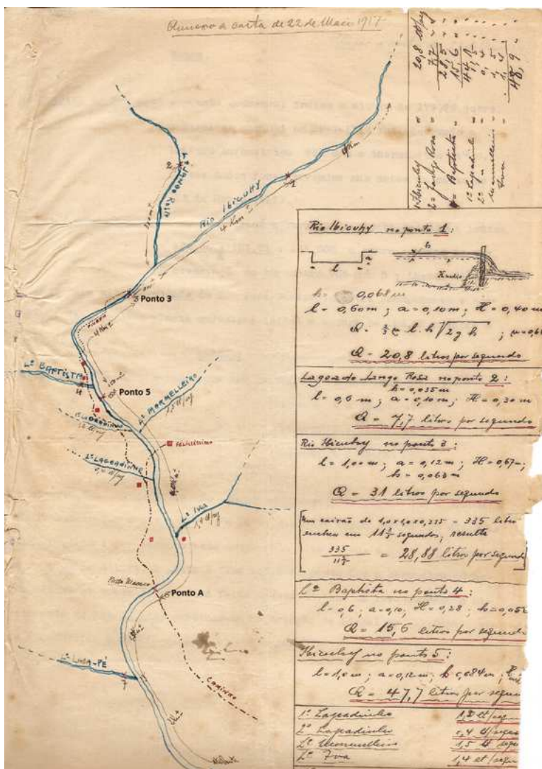
Figura 52: medições no Rio Ibicuí realizadas em 15 e 27 de abril de 1917, nos pontos 3 e 5, respectivamente. O local identificado como ponto A é o Passo do Macaco, onde a adutora foi implantada, no momento da execução do projeto, sobre o curso d'água. Pontos 3, 5 e A destacados pelo autor. Fonte: acervo da Casa de Memória Edmundo Cardoso, Coleção Astrogildo de Azevedo.
