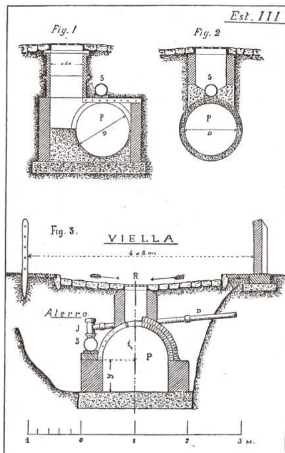
Figura 65: perfil de condutos do tipo circular para canalização do curso d'água em viela sanitária ou terreno particular com aterro. O cano "D" é o ramal de esgoto, que chega em "S", rede de esgoto que acompanha o coletor pluvial "P" alimentado pelo ralo "R". Na Fig. 3, é possível ver a região aterrada sobre a tubulação. Fonte: Brito (1943f).
