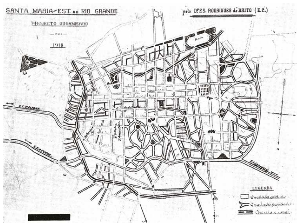
Figura 57: plano de melhoramentos de Santa Maria elaborado por Brito no ano de 1918. O norte da imagem encontra-se voltado para baixo. Fonte: Brito (1943f).
