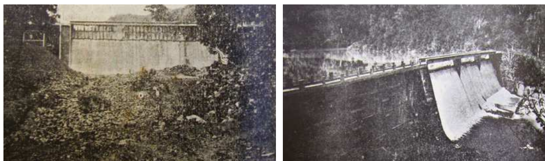
Figuras 68 e 69: barragem acumuladora vista de dois ângulos. A primeira figura é logo após a construção, com os pontalões ainda escorando a passagem por cima da queda d'água. A segunda, é a barragem já concluída. Presume-se que os anos das fotos sejam os mesmos das publicações. Fontes: Revista CCA (1931) e Abreu (1953), respectivamente.
