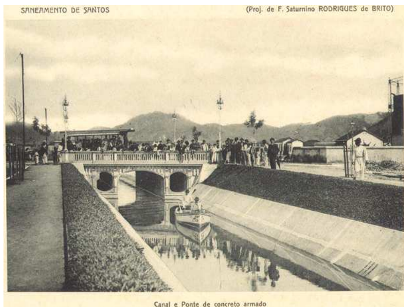
Figura 03: ponte na Av. C. Nebias em concreto armado. Fonte: Brito (1943d).
