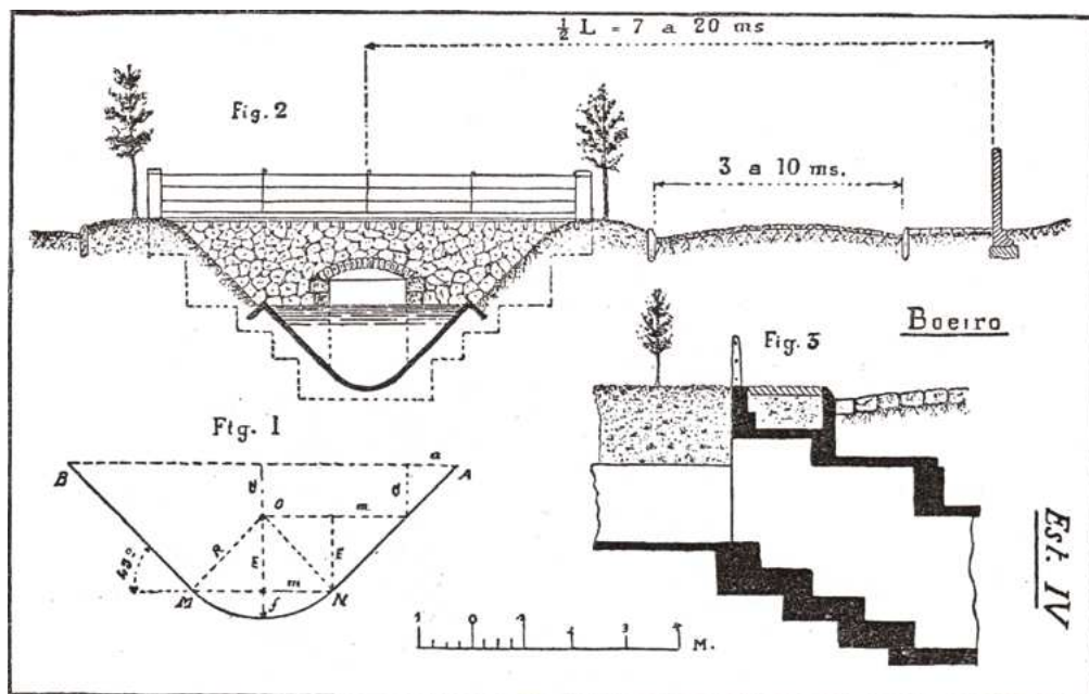
Figura 64: perfil e estudos da avenida canal no projeto de saneamento de Santa Maria. Fonte: Brito (1943f).
