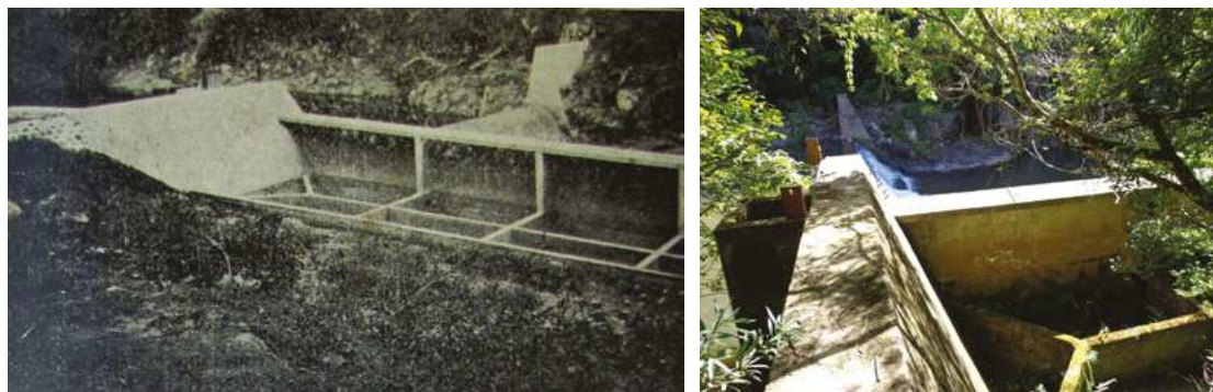
Figuras 72 e 73: a primeira figura é a represa de tomada com os tanques de sedimentação, primeira etapa do tratamento d'água antes de entrar para a adutora. A segunda é a represa, em 2012, já desativada devido à construção da barragem em Val de Serra. Fontes: Revista CCA (1931) e foto do autor em 2012, respectivamente.
