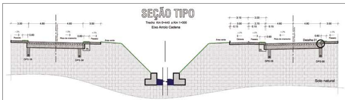
Figura 103: corte transversal de parte da Av. Dom Ivo Lorscheiter. Fonte: Programa de Aceleração do Crescimento (PAC), Prefeitura Municipal de Santa Maria.
